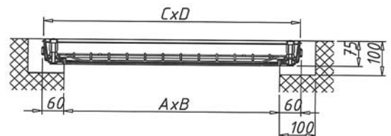
aluminium hauteur de remplissage 68 mm
